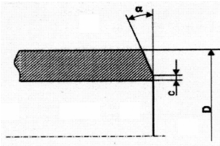
Рис. 1 – угол скоса кромки трубы
